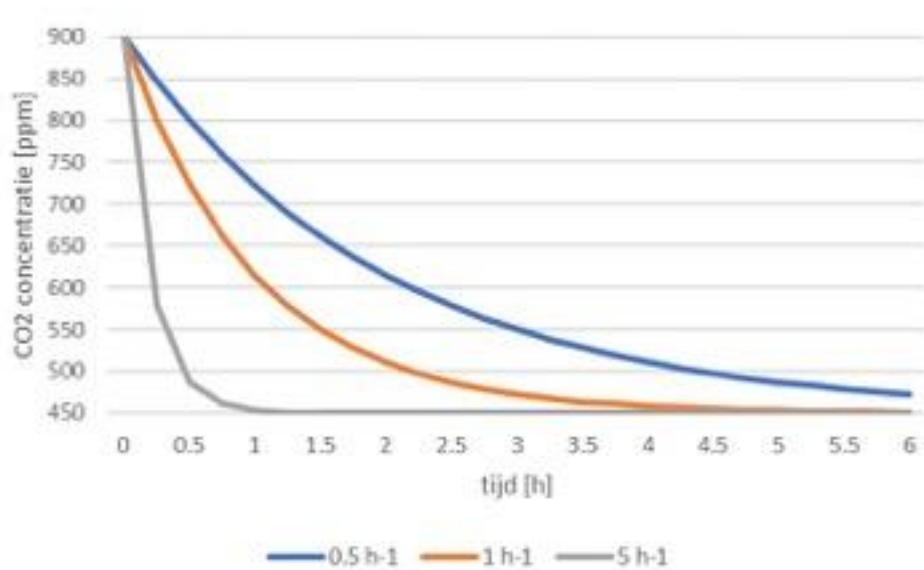
Afbeelding B9.1: Verloop van de CO 2 -concentratie bij verschillende waarden voor het ventilatievoud ( C_0 = 450 ppm, C_{\text{eind}} = 900 ppm).
