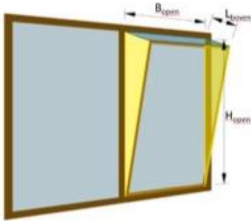
Afbeelding B6.1: Grafische weergave maten bij een kiepraam.
